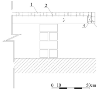
DETAY AÇILIMI
